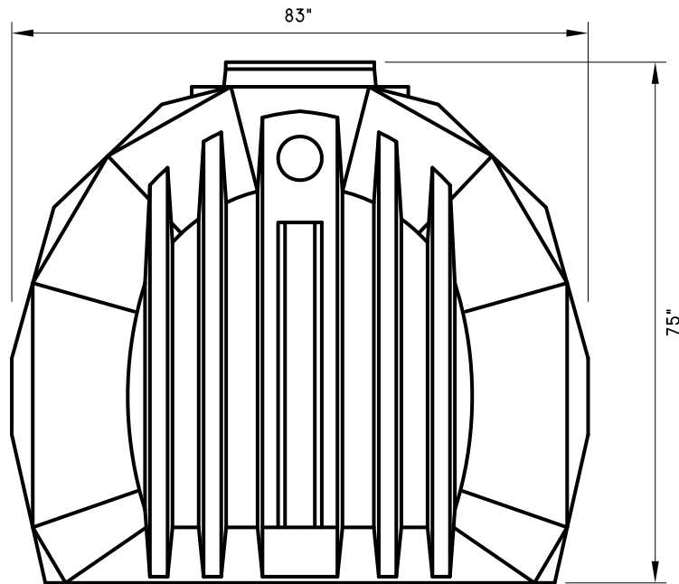
END ELEVATION
