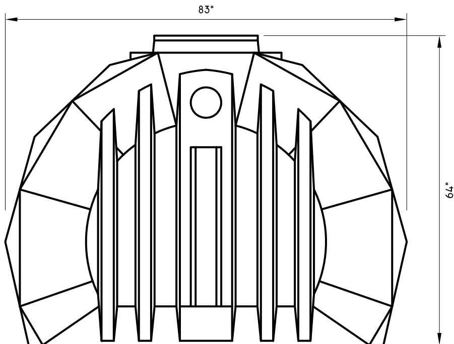
END ELEVATION
