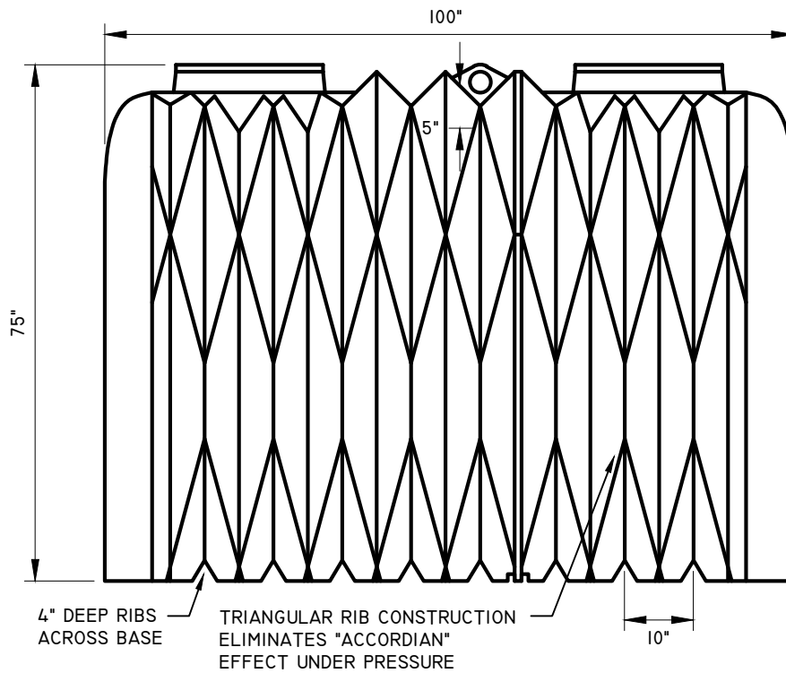
ELEVATION
