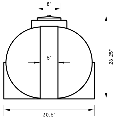
END ELEVATION
