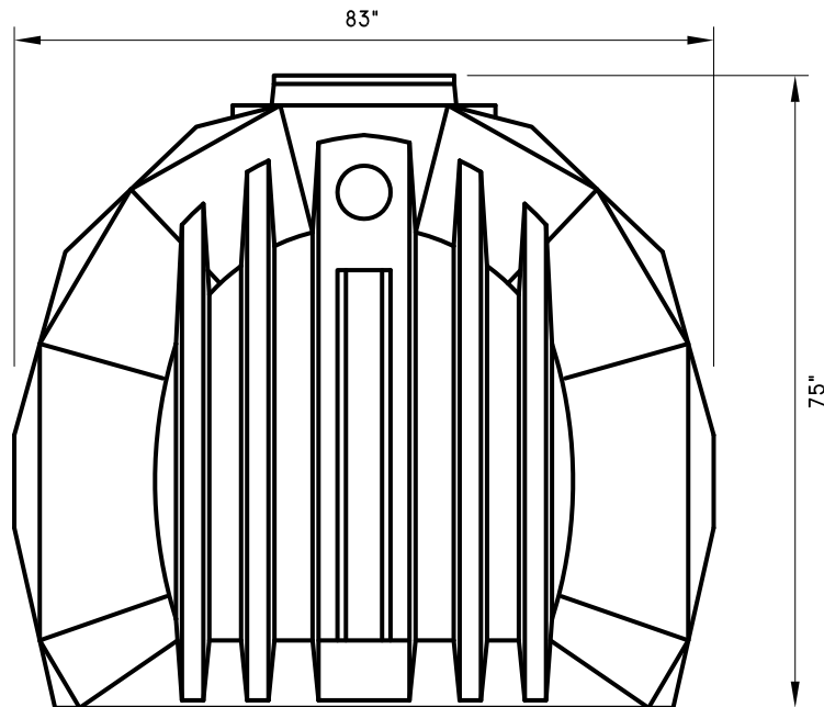
END ELEVATION
