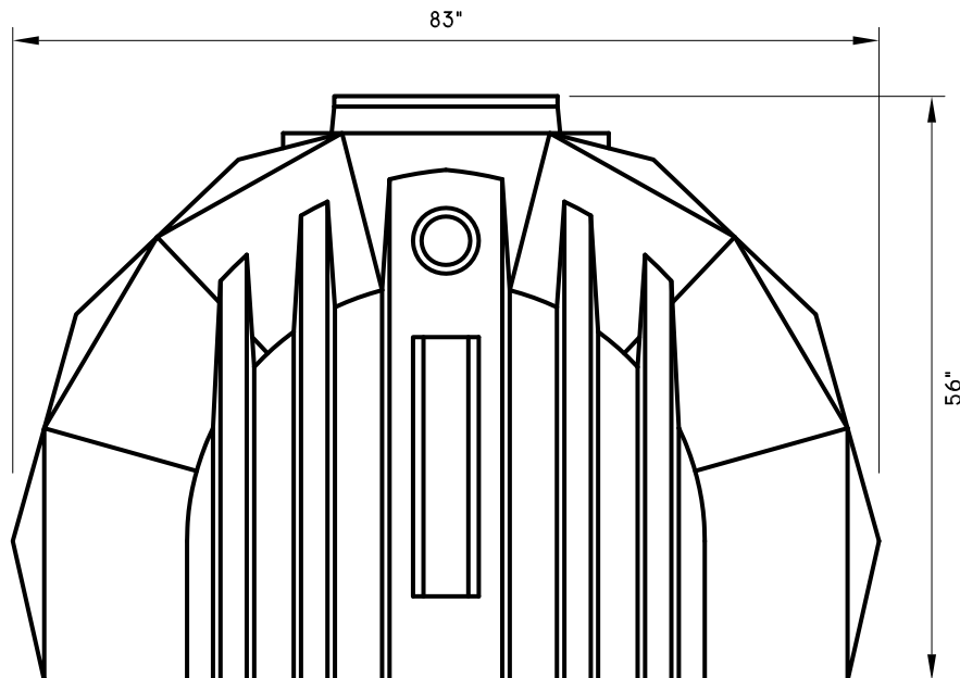
END ELEVATION
